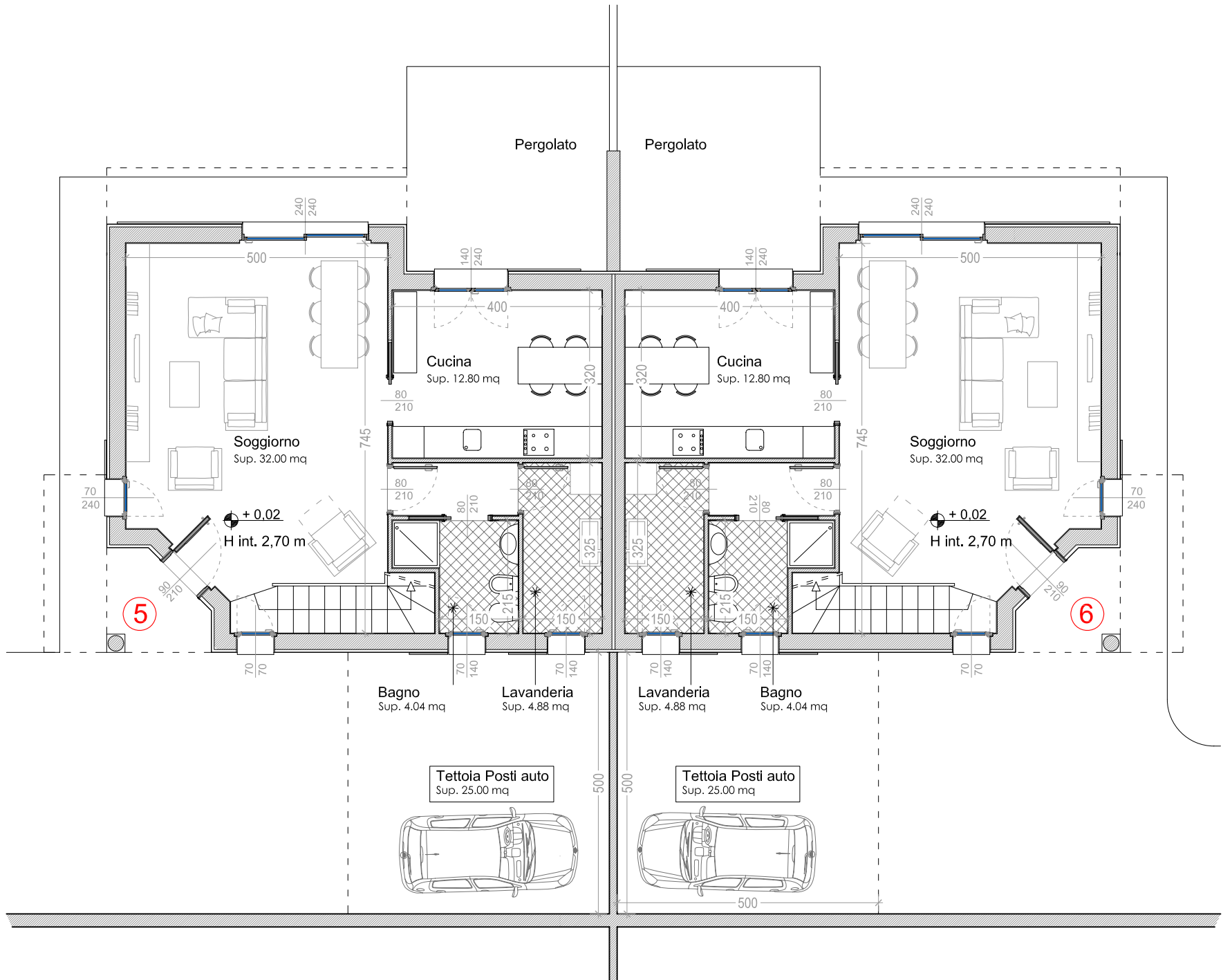
PIANTA PIANO TERRA - Villette n. 5 - 6
