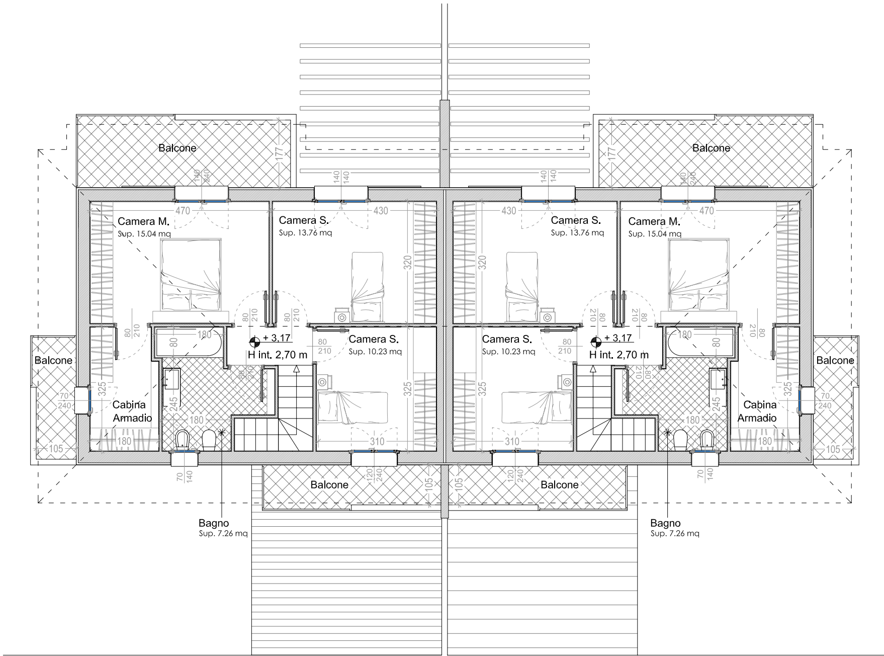
PIANTA PIANO PRIMO - Villetta n. 5 - 6
