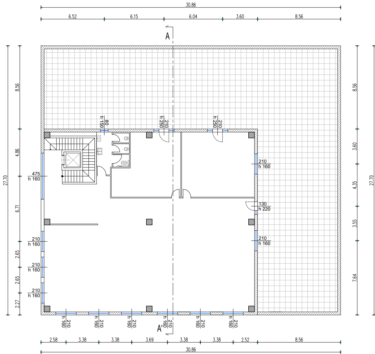
PIANTA PIANO PRIMO scala 1:200
