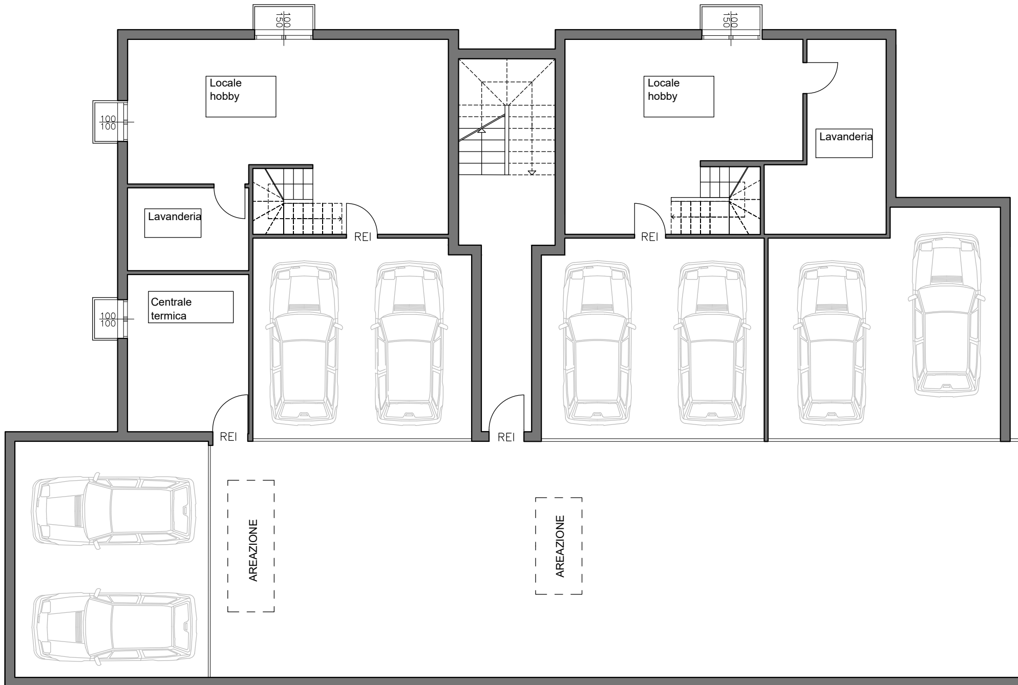
PIANTA PIANO INTERRATO scala 1:100
